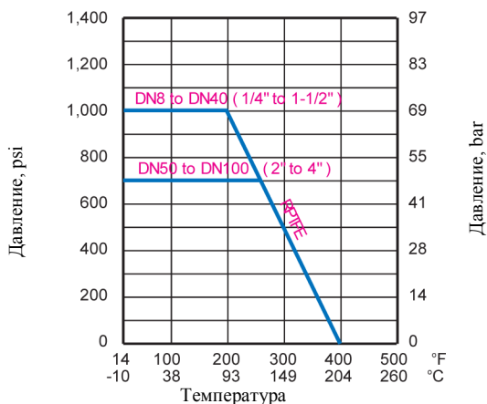
График: давление/температура
